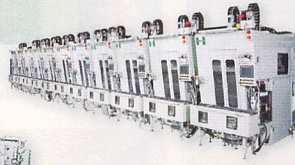
ミッションケース加工FTLライン
